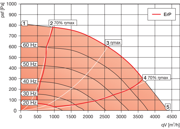
KCF-N 355 D4 40
