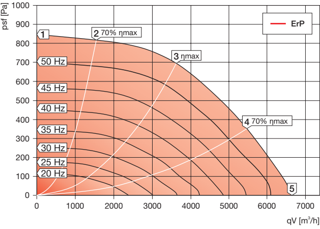
KCF-N 450 D4 40
