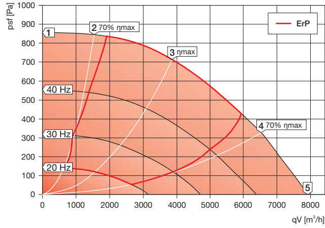
KCF-N 500 D4 40
