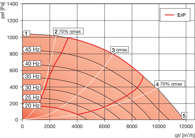
KCF-N 560 D4 40
