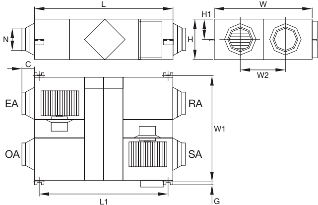
■ CHRU-TF 150 - CHRU-TF 650
