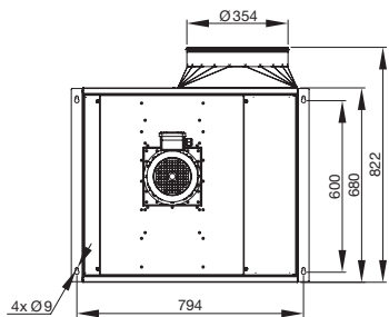
■ KCX 355 D430
