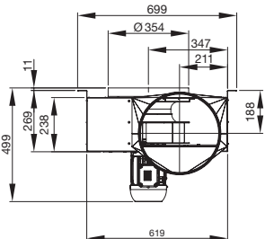
■ KCX 315 D430
