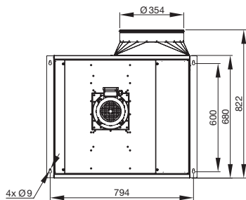
■ KCX 315 D430
