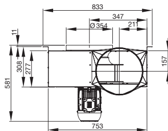
■ KCX 450 D430
