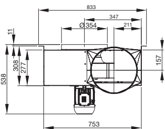
■ KCX 400 D430
