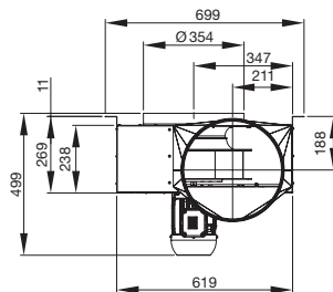
■ KCX 355 D430
